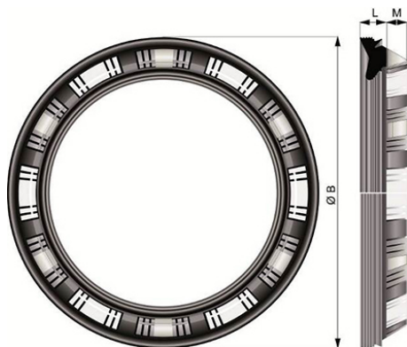
DN75-125
